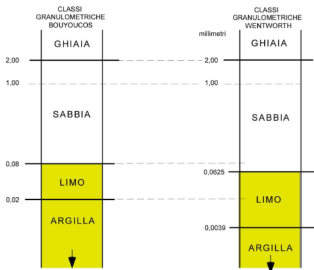
Fig. 1 - Confronto tra le scale granulometriche di Bouyoucos e di Wentworth.
