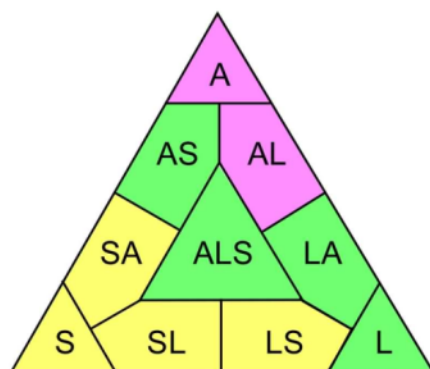
Fig. 3 - Il triangolo di Shepard per l'associazione tessitura-permeabilità
