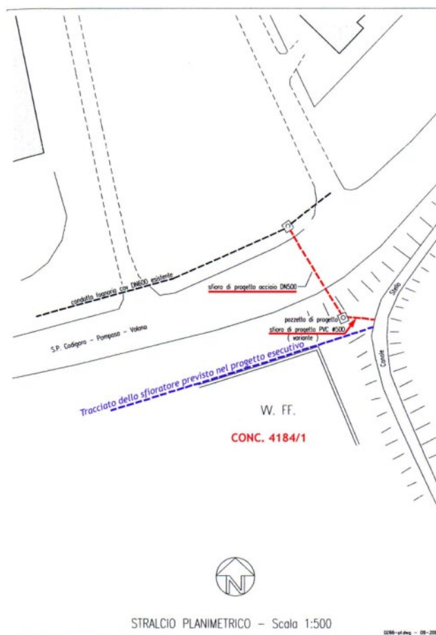
Fig. 10 (a destra) - Planimetria del punto di scarico di troppo pieno nel Canale Stella (punto n.2 della cartografia).
