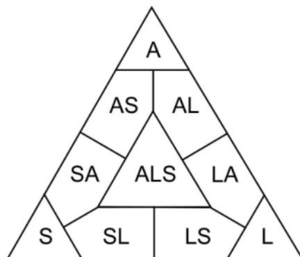
Fig. 2 - Il triangolo di Shepard per classificazione dei tipi litologici con granuli inferiori a 2 mm di diametro.
