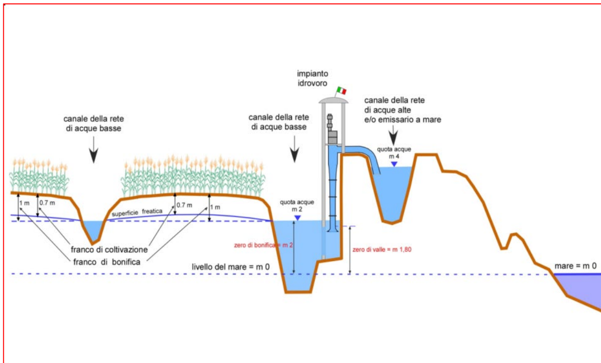
Schema di rapporti altimetrici fra acque superficiali e superficie freatica
