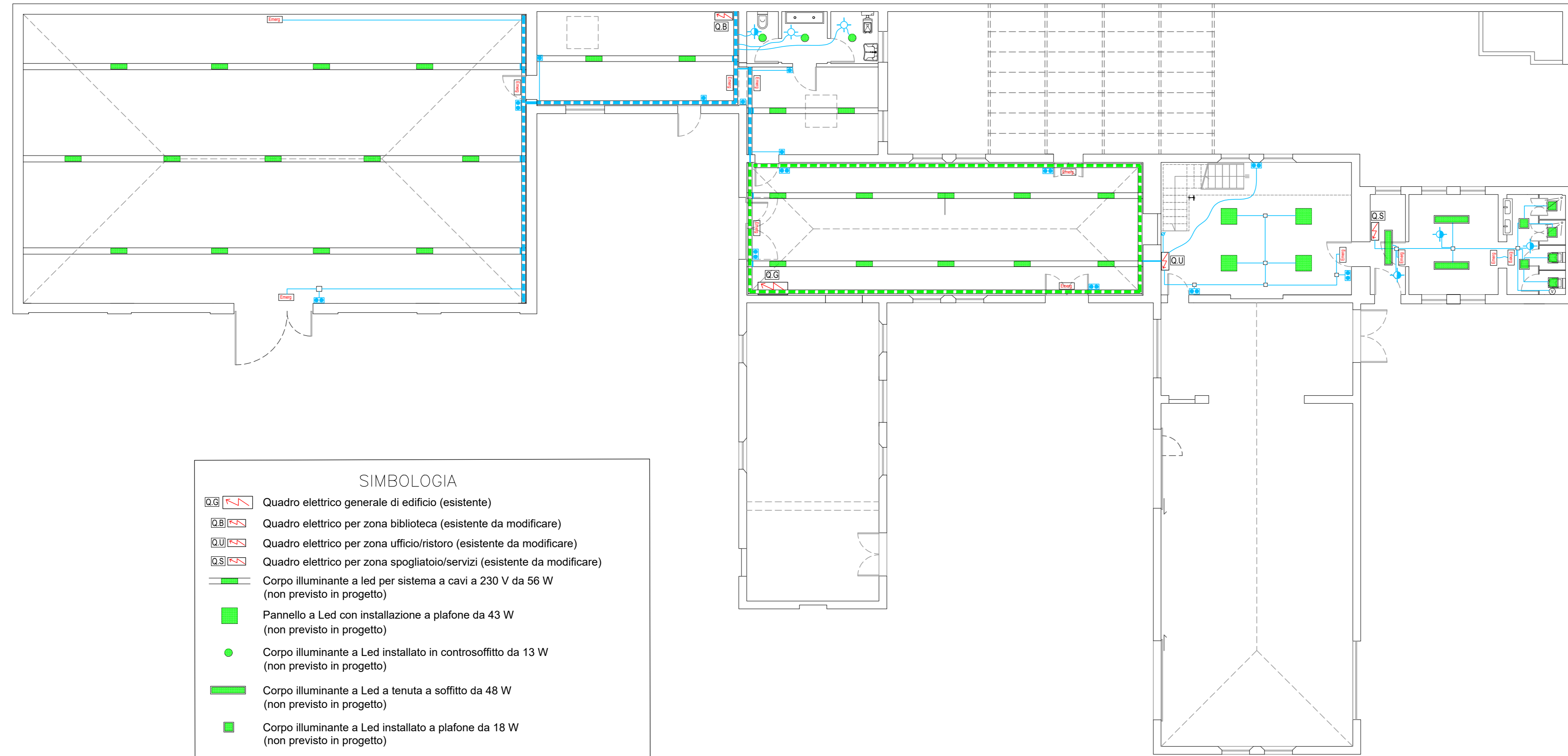
PIANTA SOPPALCO
