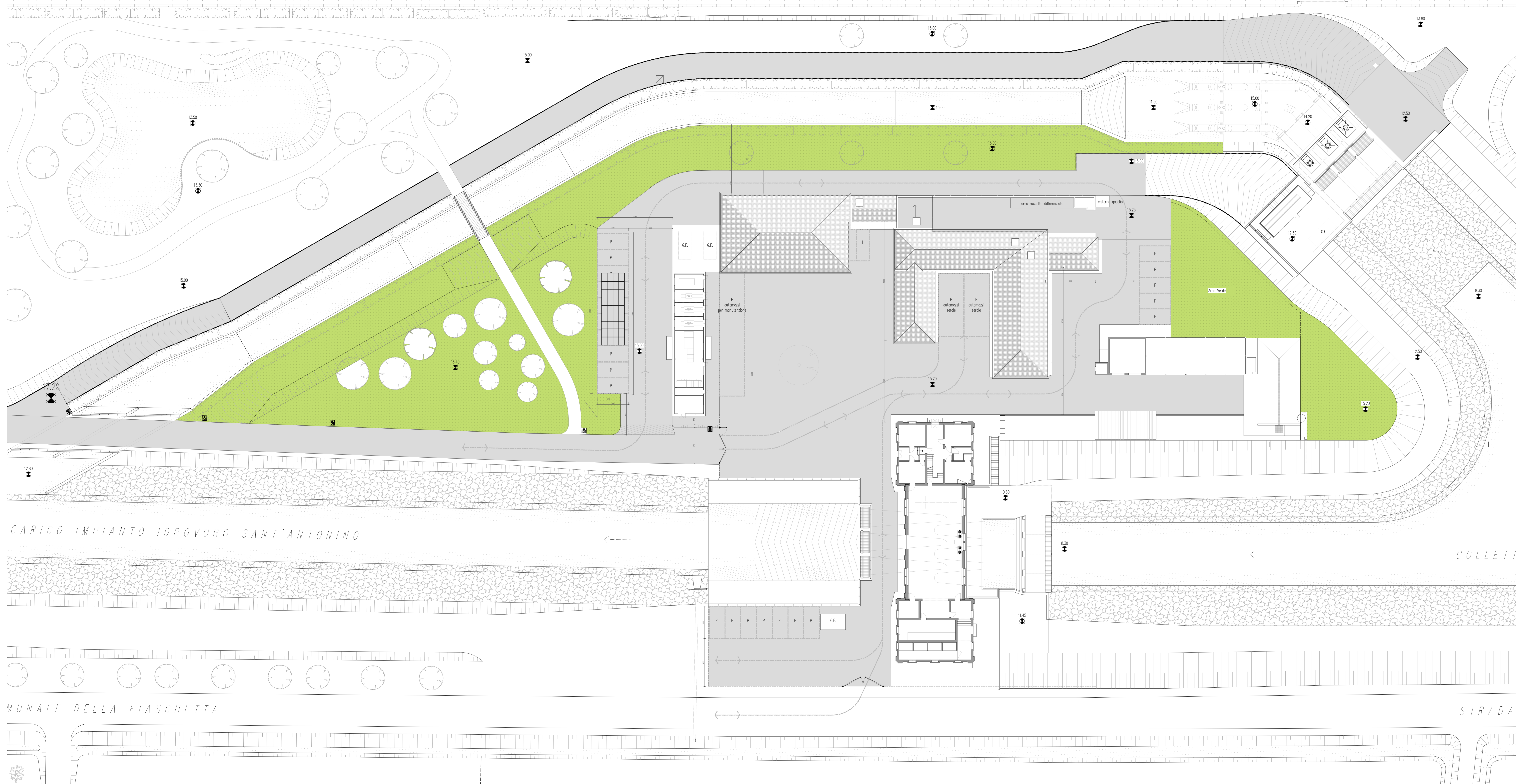
Planimetria generale Scala 1:200
