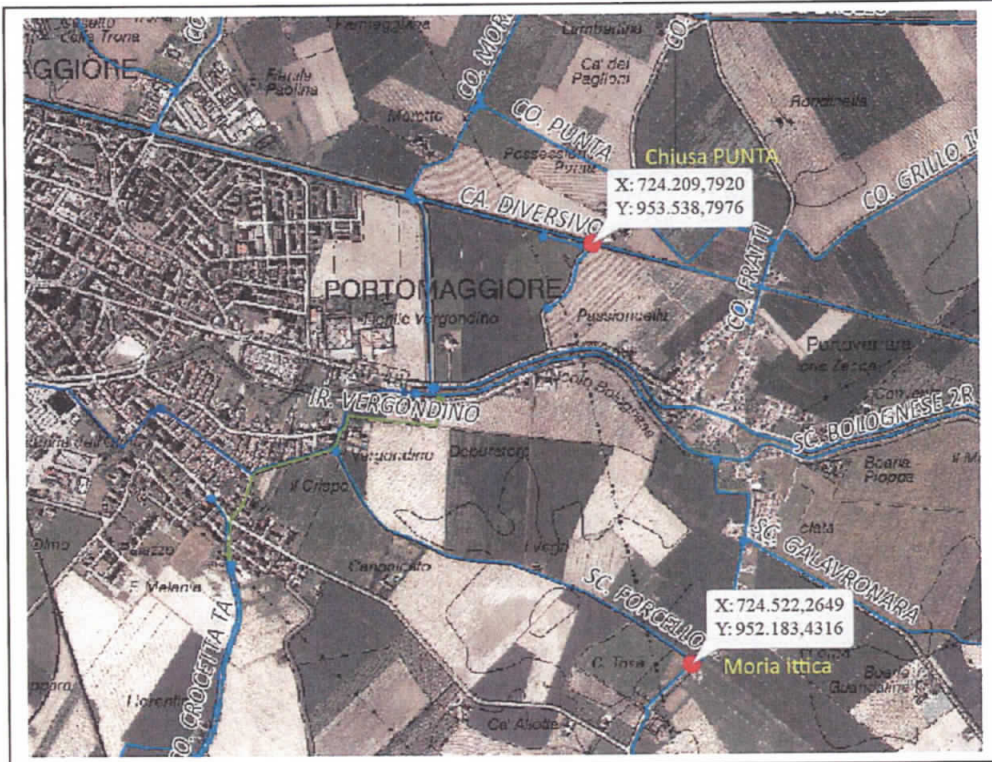
Chiusa Punta lungo Via Paglioni con le tre paratoie automatizzate
