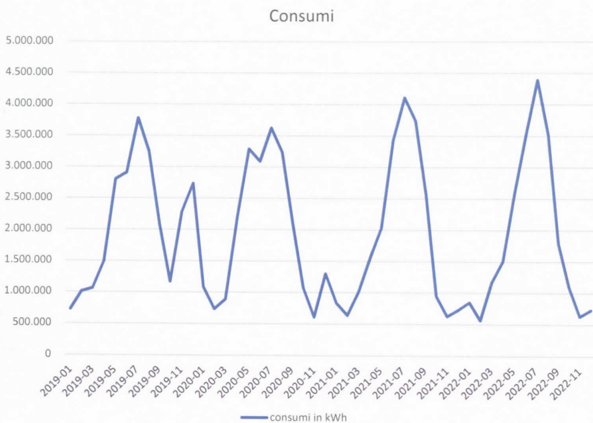
Grafico n. 5 – Consumo in kWh degli impianti negli anni 2019-20-21-22
