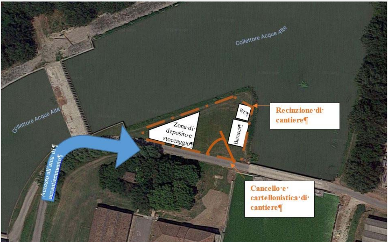
Figura 10. Planimetria area di accantieramento.
