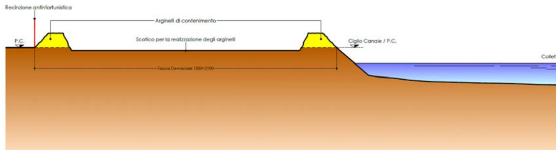
Figura 5. Sezione trasversale tipo dell'area di contenimento.
