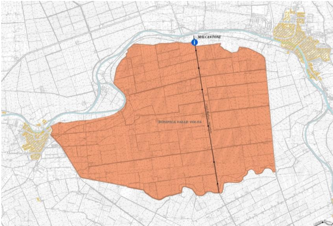
Il Bacino principale Valle Volta con l'Impianto Idrovorio Malcantone.
