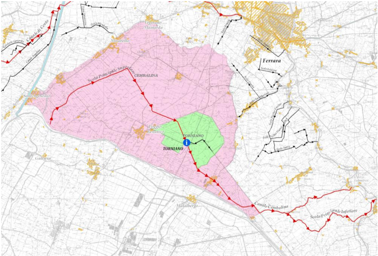
Il Bacino principale Cembalina, con il sottobacino Torniano e il relativo Impianto Idrovoro.
