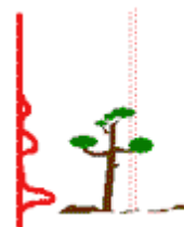
Punti riflessi lungo un profilo lidar. Il raggio laser penetra la vegetazione, se non eccessivamente densa, e riflette quindi punti a vari livelli.
