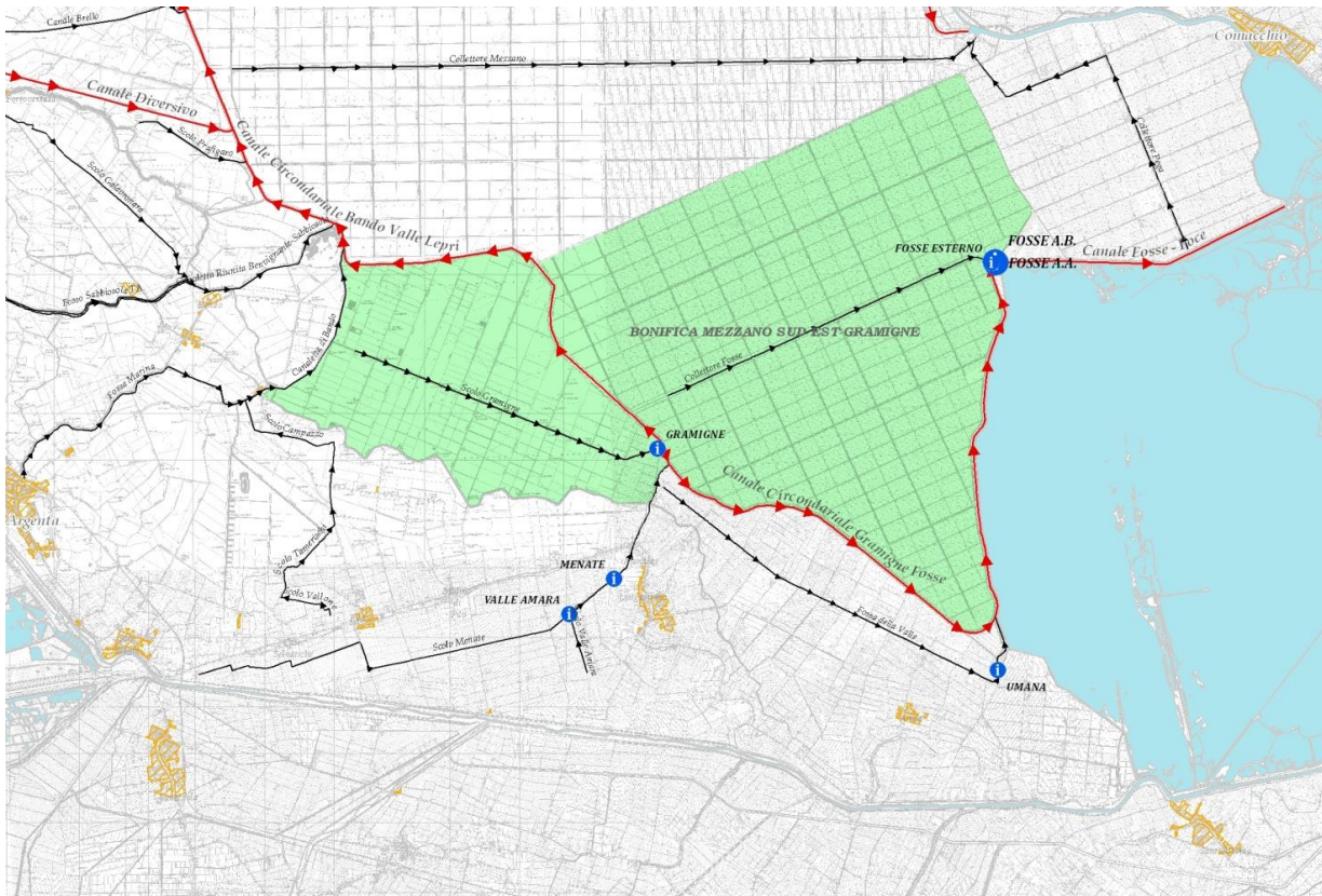
Il Bacino principale Mezzano Sud-Est Gramigne, con gli Impianti Idrovori Gramigne, Fosse Acque Basse e Fosse Acque Alte.
