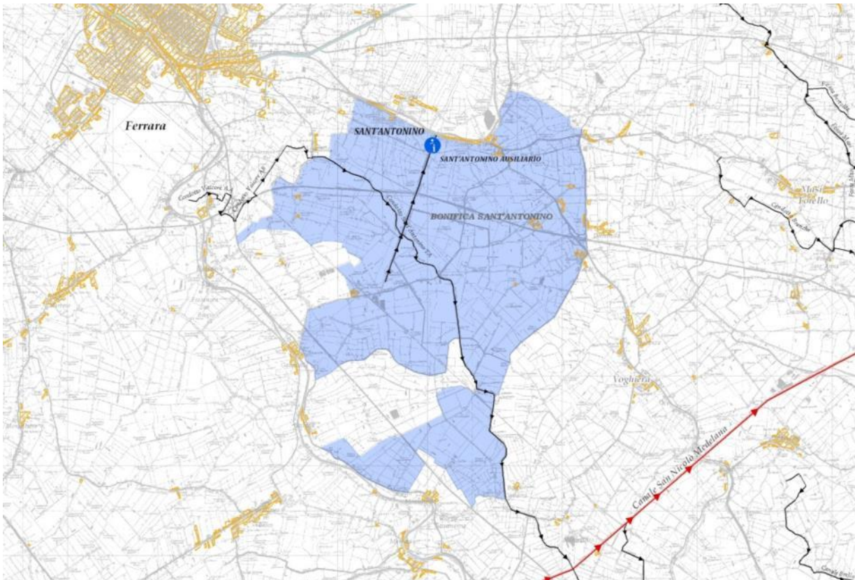
Il Bacino principale Bonifica di S. Antonino e relativo Impianto Idrovorio.
