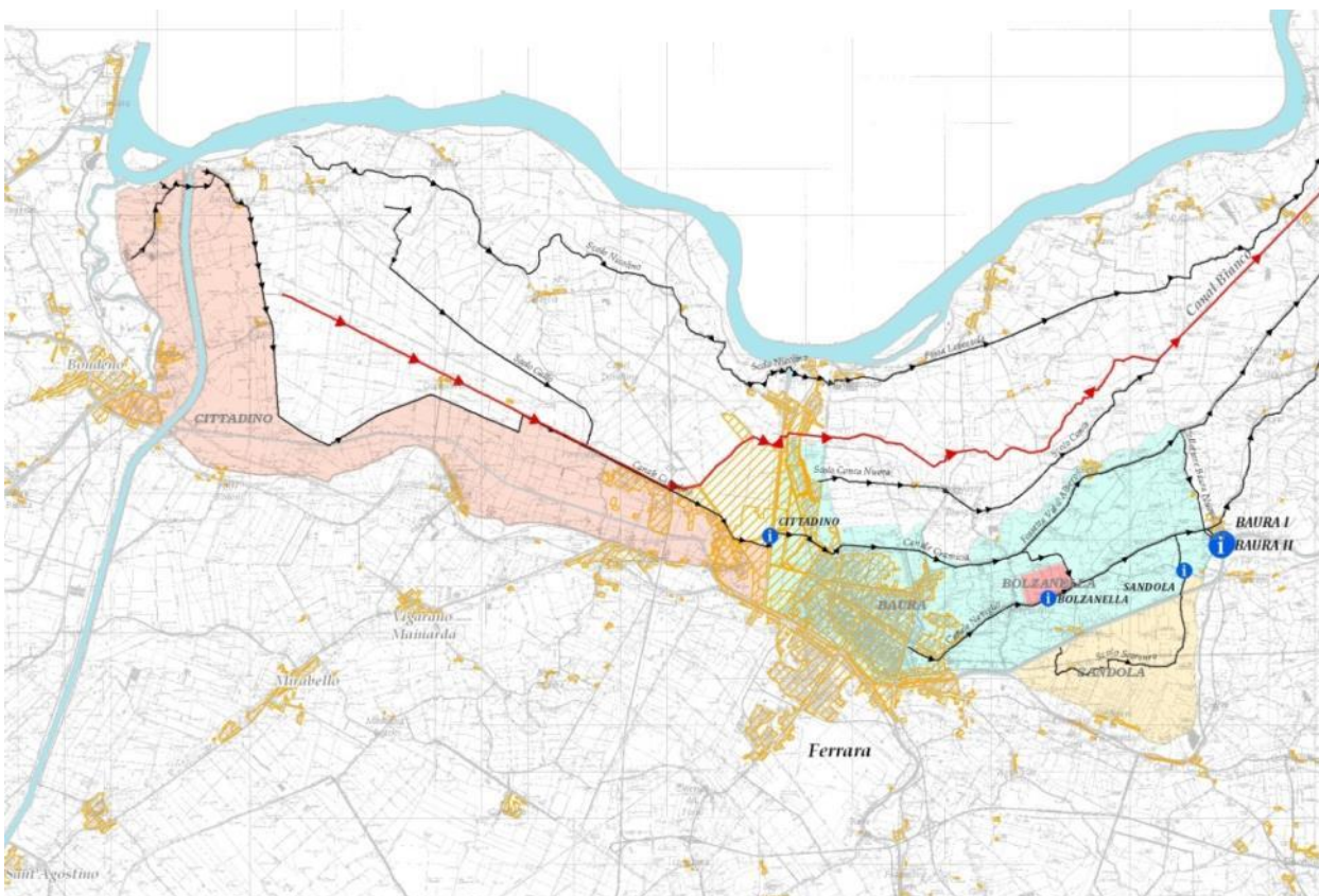
Il Bacino principale Baura, sottobacini e impianti idrovori. Sotto, veduta aerea degli impianti di Baùra.
