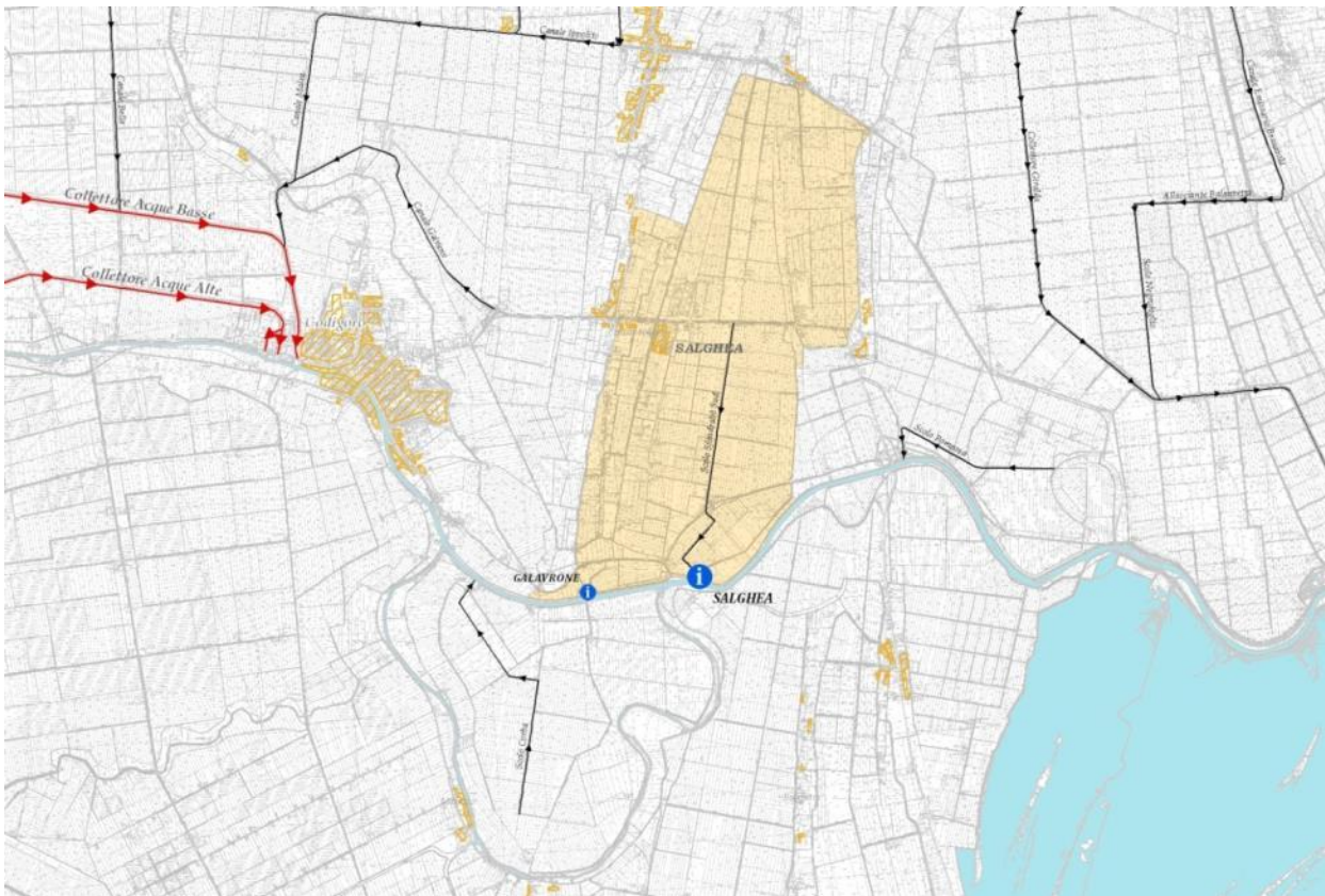
Figura a sinistra: Impianto Idrovaro Campello.
