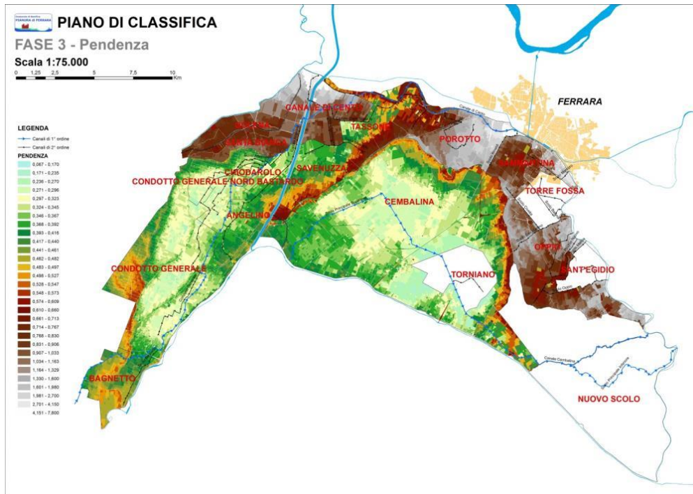
Elaborazione della pendenza dei terreni rispetto ai recapiti in acque esterne. Le tonalità più chiare rappresentano le zone di minor pendenza.
