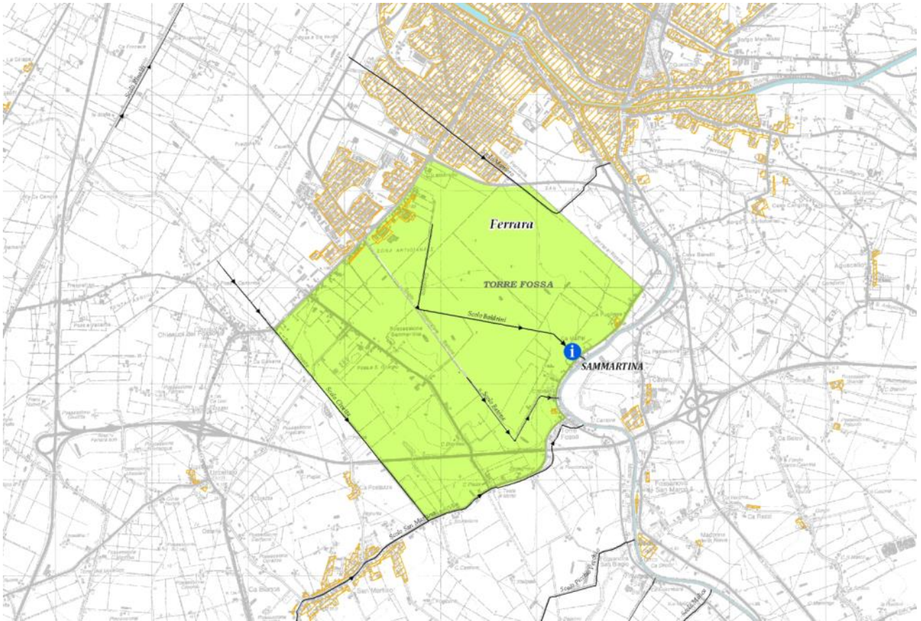
Il Bacino principale di Torre Fossa, con relativo Impianto Idrovo Sammartina
