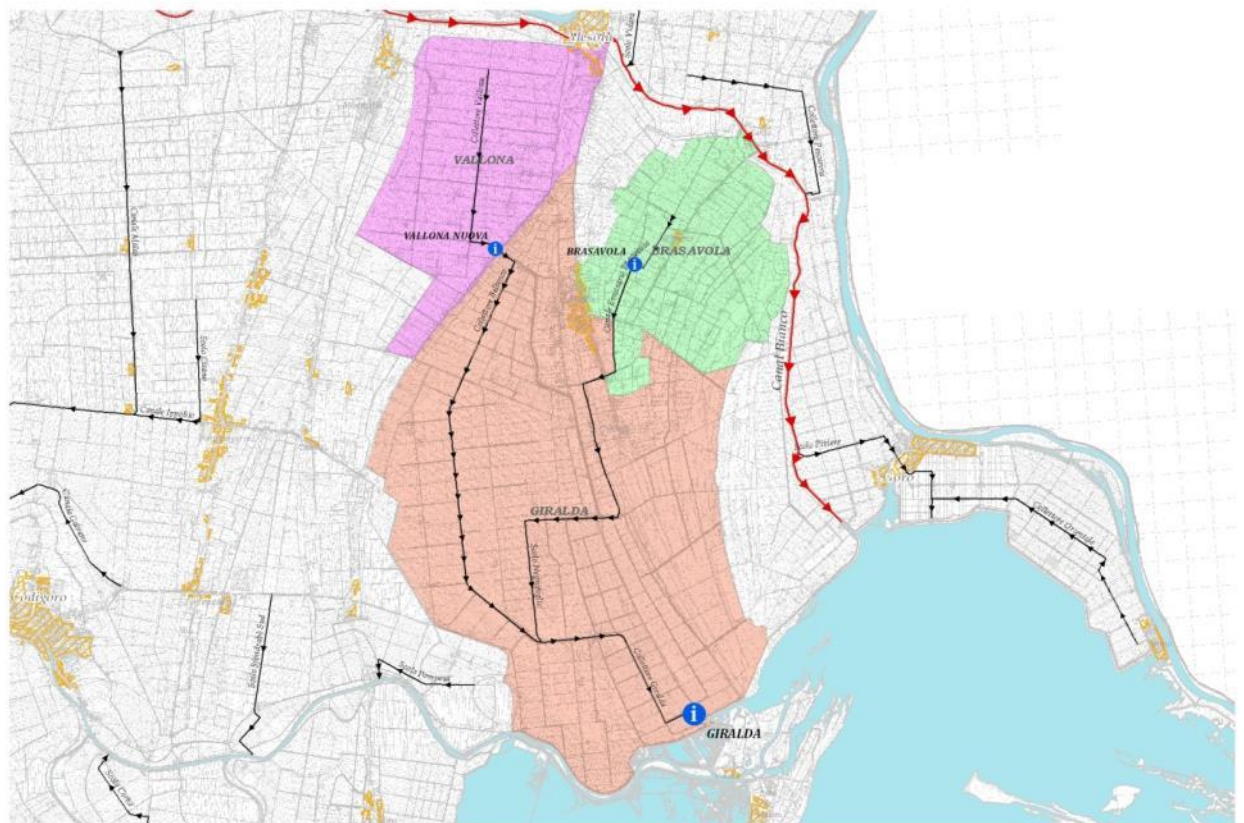
Il Bacino principale Giralda, sottobacini e impianti idrovori.
