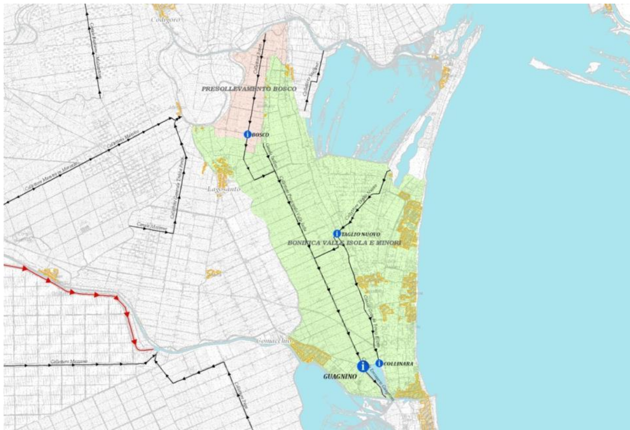
Il Bacino principale Valle Isola e minori, relativi sottobacini e impianti idrovori.
