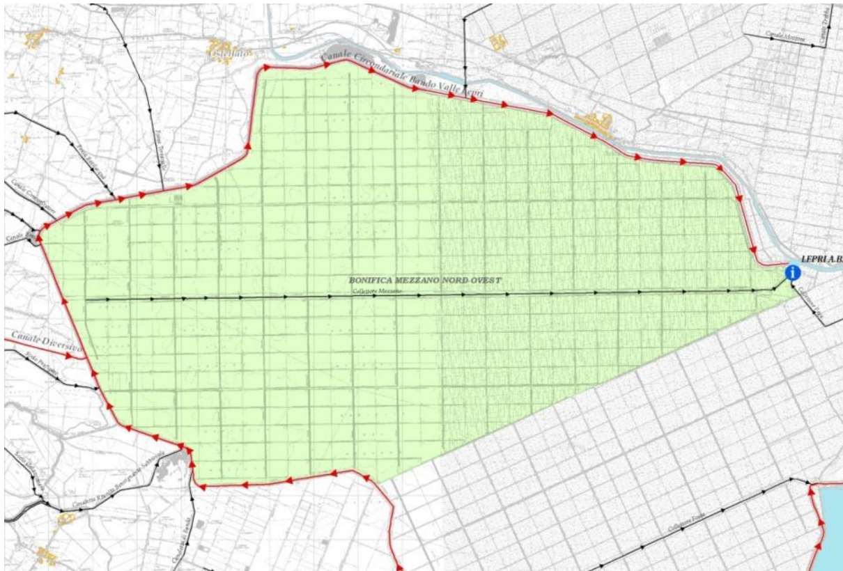
Il Bacino principale Mezzano Nord-Ovest e relativo Impianto Idrovo Lepri Acque Basse Mezzano.
