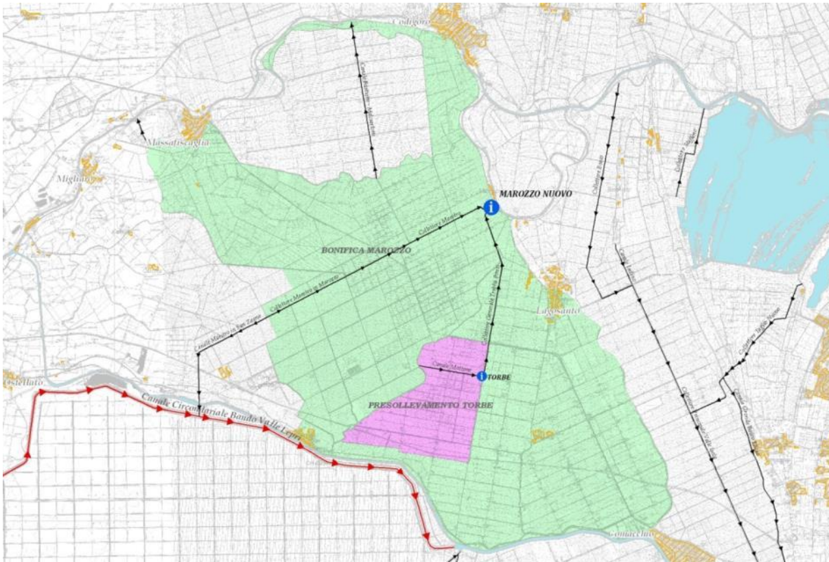
Il Bacino principale Marozzo e il relativo Impianto Idrovoro Nuovo Marozzo e l'impianto idovoro di presollevarmento Torbe.
