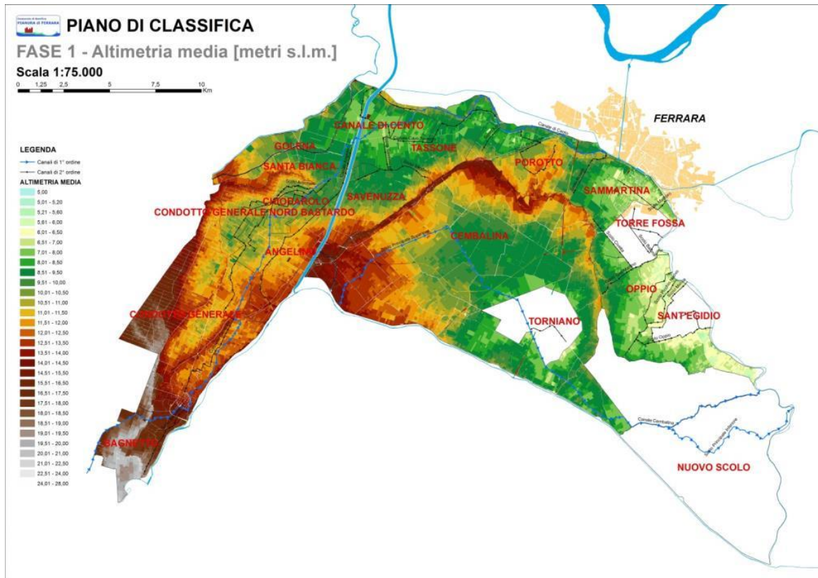
Rappresentazione altimetrica ottenuta attraverso l'elaborazione delle particelle catastali. Le aree non colorate corrispondono a sottobacini a sollevamento meccanico.
