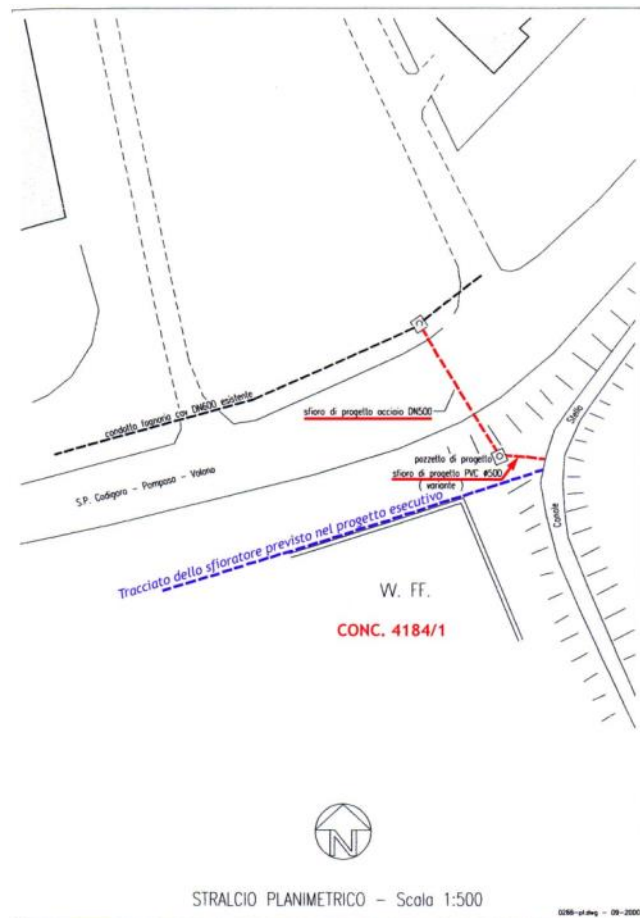
Fig. 10 (a destra) - Planimetria del punto di scarico di troppo pieno nel Canale Stella (punto n.2 della cartografia).
